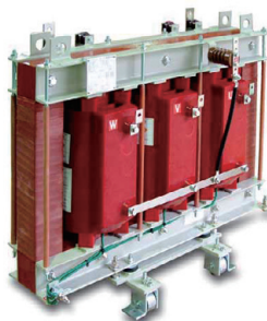
▲発電機用接地変圧器
