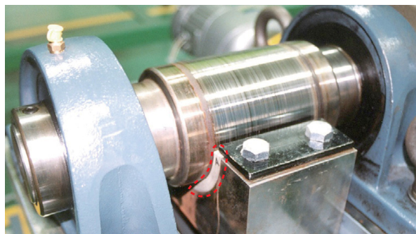
赤枠の部分が試験片。高い荷重(10N/mm 2 )をかけた際の耐摩耗性を評価
